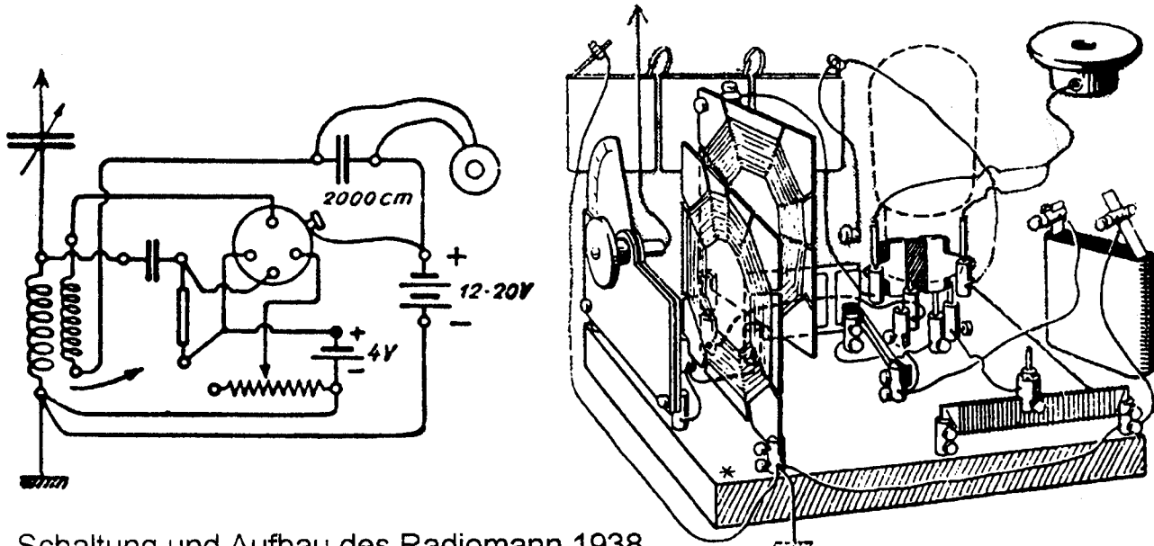
Schaltung und Aufbau des Radiomann 1938
